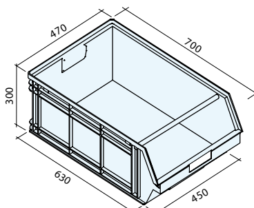
Art. PL8951 (OP-5Z) (con travesaño) Dim. 700/630x450x300h mm Cap. 88 litros
