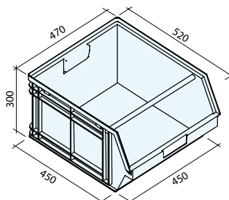
Art. PL8151 (OP-5P4Z) (con travesaño) Dim. 520/450x450x300h mm Cap. 63 litros
