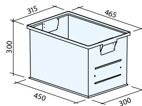
Art. PJ7351 (TR-4A5) 450x300x300h mm. Cap. 40,5 litros
