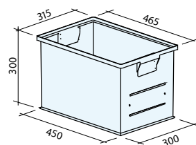
Art. PJ7351 (TR-4A5) 450x300x300h mm. Cap. 40,5 litros
