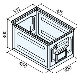
Art. LA7320 (TRM-4A5) Dim. 450x300x300h mm Cap. 40,5 litros
