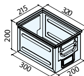
Art. LA4120 (TRM-3) Dim. 300x200x200h mm Cap. 12 litros
