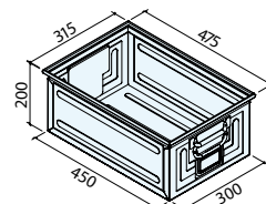
Art. LA6520 (TRM-4) Dim. 450x300x200h mm Cap. 27 litros
