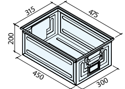
Art. LA6520 (TRM-4) Dim. 450x300x200h mm Cap. 27 litros
