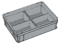
Art. PP6551 (CE-623) Dim 357x278x90h mm
