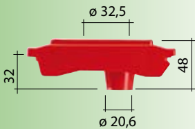
Art. NC9510 (NC 301) / ISO 30 Dim. 65x138x48h mm
