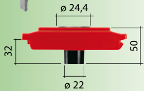
CONO MORSE 3 Art. NC9730 (NC 347) Dim. 64x138x50h mm
