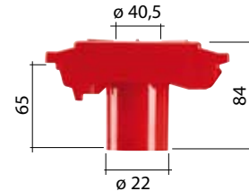
Art. NC9570 (NC 307) / VDI 40 Dim. 83x138x82h mm
