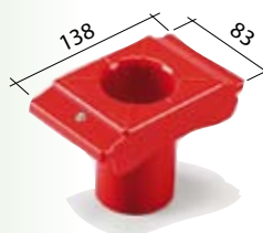
Art. NC9580 (NC 308) / VDI 50 Dim. 83x138x98h mm
